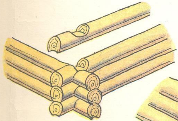
в обло (с остатком)
