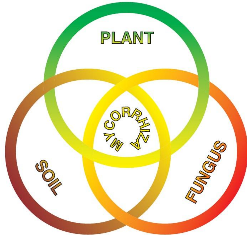
Рис.1. Схема взаимосвязи микоризных грибов, растений и почвы (Brundrett, 2008)
