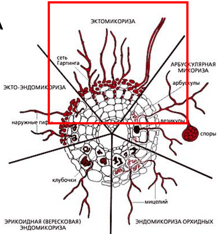
Рис.2. Морфологические особенности различных типов микоризы. В центре – поперечный срез корня. (Дьяков, 2003)
