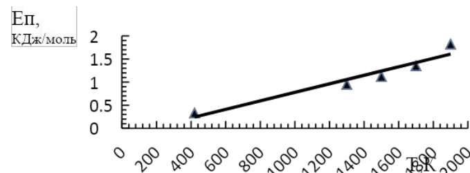
Рис. 4 Зависимость пространственной энергии E_p углеродного слоя C_{106} от температуры
