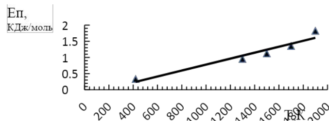
Рис. 4 Зависимость пространственной энергии E_n углеродного слоя C_{106} от температуры
