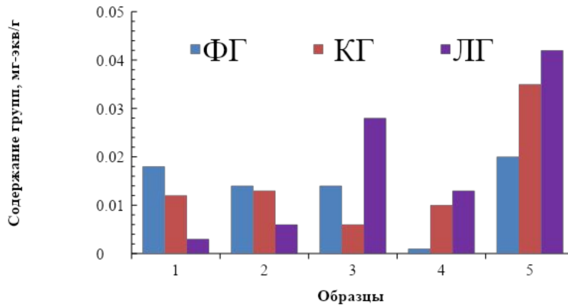
Рис. 8 Функциональный состав окисленных образцов ТУ
