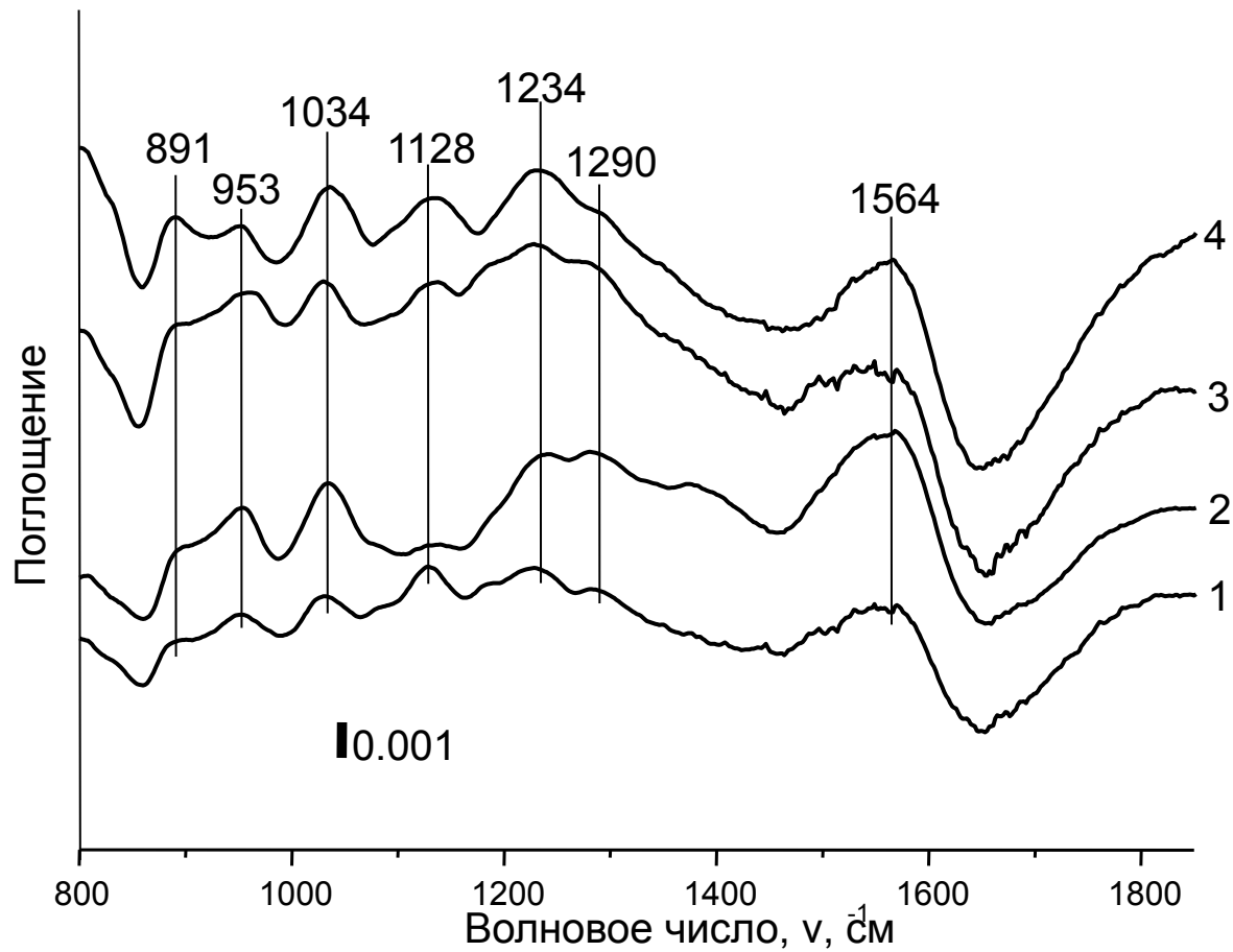
Рис. 7 ИК спектры окисленных образцов: N 326 исходного (1) и окисленных пероксидом водорода (2), озоном (3) и кислородом ^1\text{O}_2 (4)
