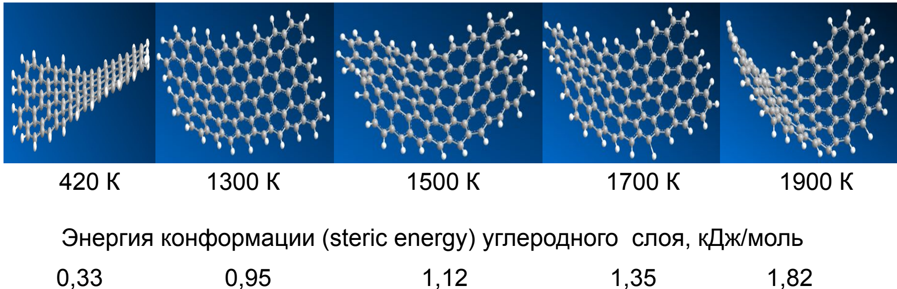
Рис. 3 Влияние заданной температуры на деформацию углеродных слоев
