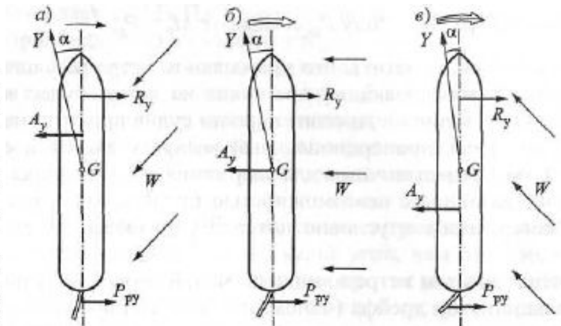
Рис. 2.10. Силы и моменты, действующие на судно в зависимости от курсового угла кажущегося ветра: а) q_w = 45^\circ ; б) q_w = 90^\circ ; в) q_w = 135^\circ
