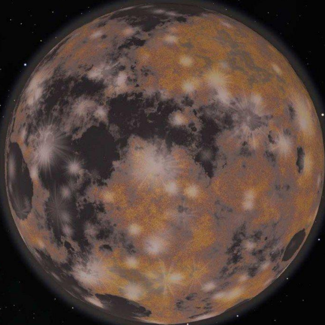
Плутон
