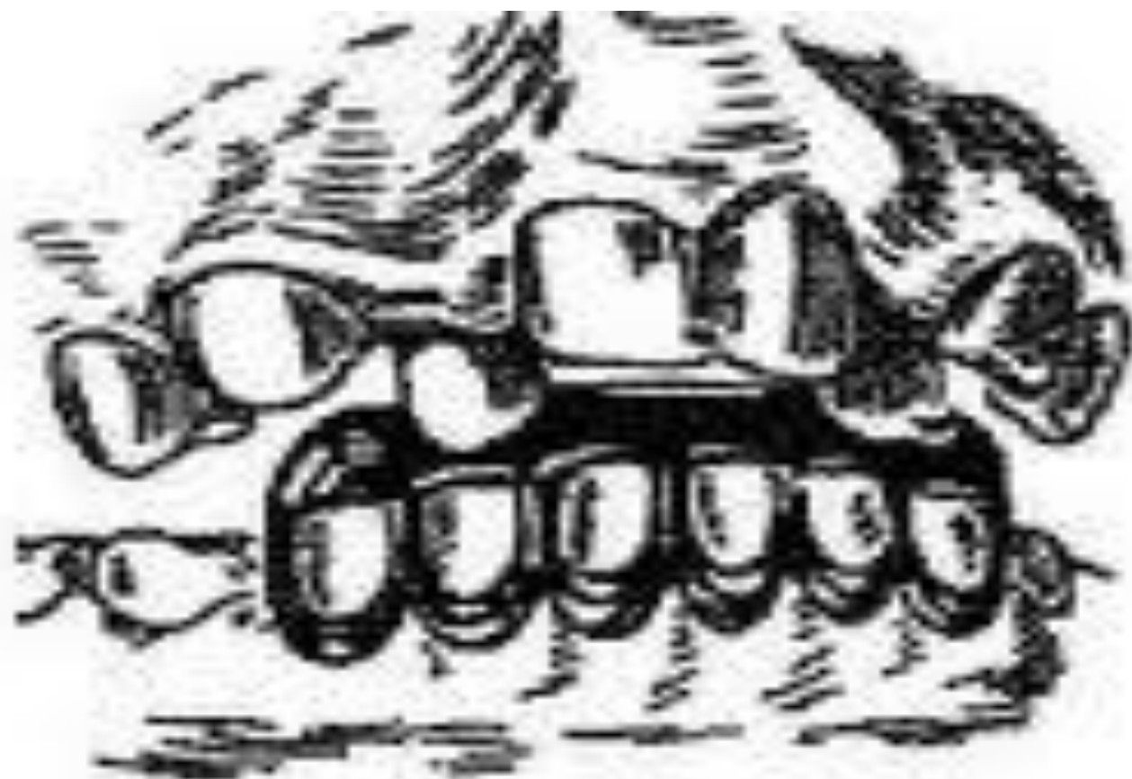
Рис. 41. Каппа Шварца
