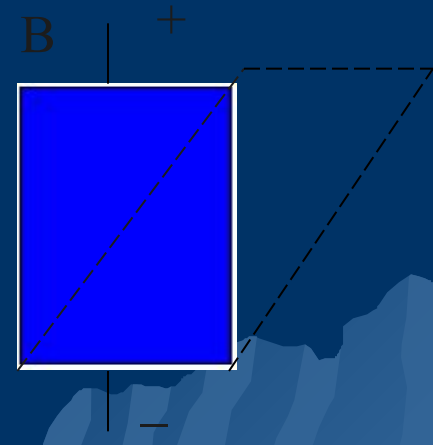
Рис. 1.10. Виды деформации пьезоэлементов: А – изменение формы элемента при продольной деформации; В - изменение формы элемента при сдвиговой деформации
