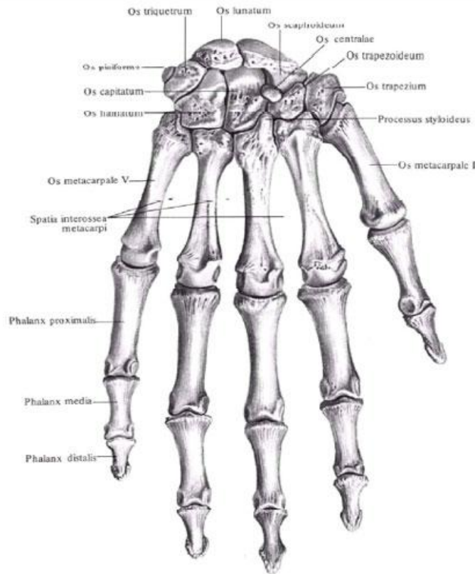
Кости кисти, ossa manus; правой (тыльная поверхность)
