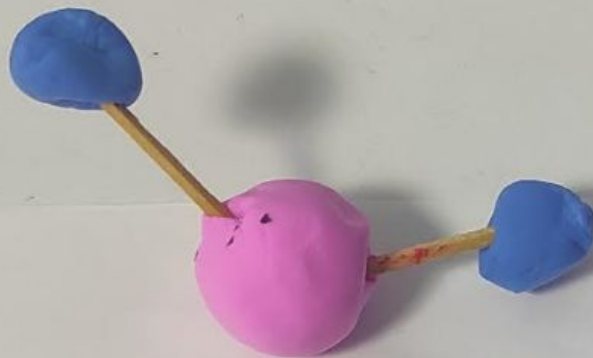
Молекула води H_2O
