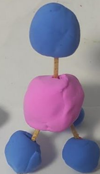
Молекула метану CH_4
