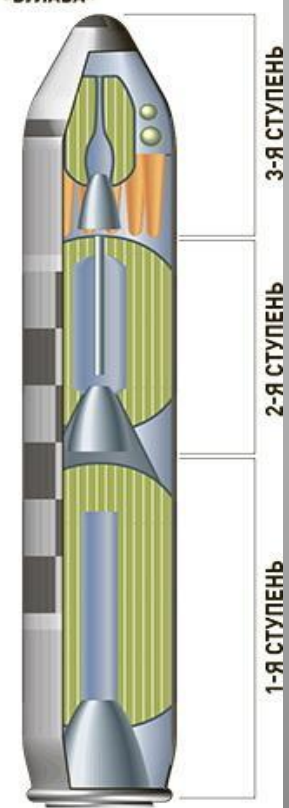
БАЛЛИСТИЧЕСКАЯ РАКЕТА МОРСКОГО БАЗИРОВАНИЯ «БУЛАВА»
