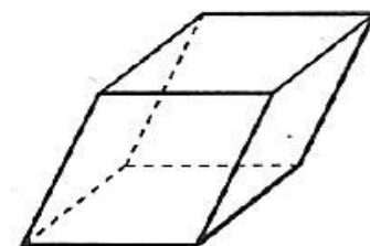
параллелепипед
