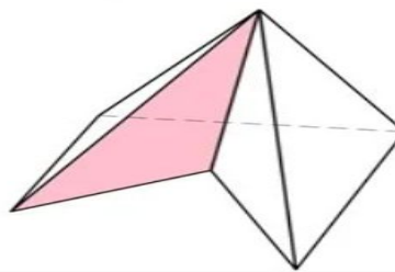
Невыпуклый многогранник
