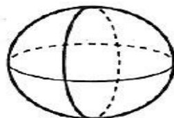
шар
