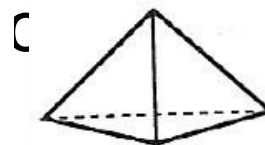
пирамида
