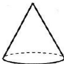
конус
