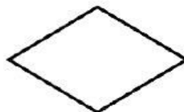
ромб
