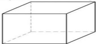
Выпуклый многогранник
