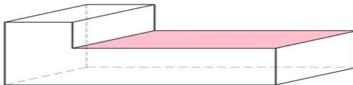
Невыпуклый многогранник
