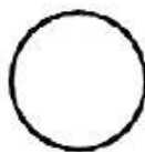
круг
