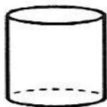
цилиндр
