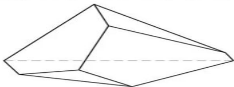
Выпуклый многогранник
