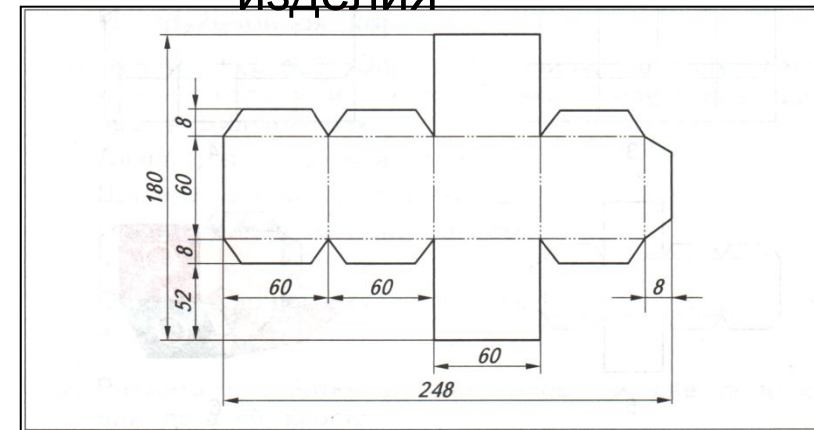
чертёж изделия
