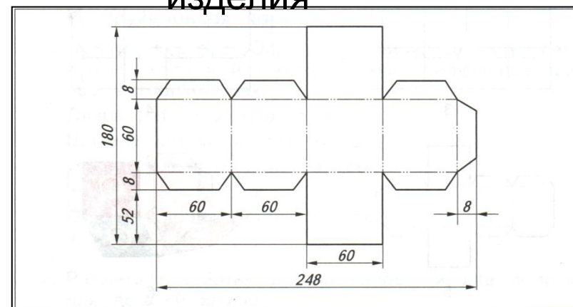
чертёж изделия
