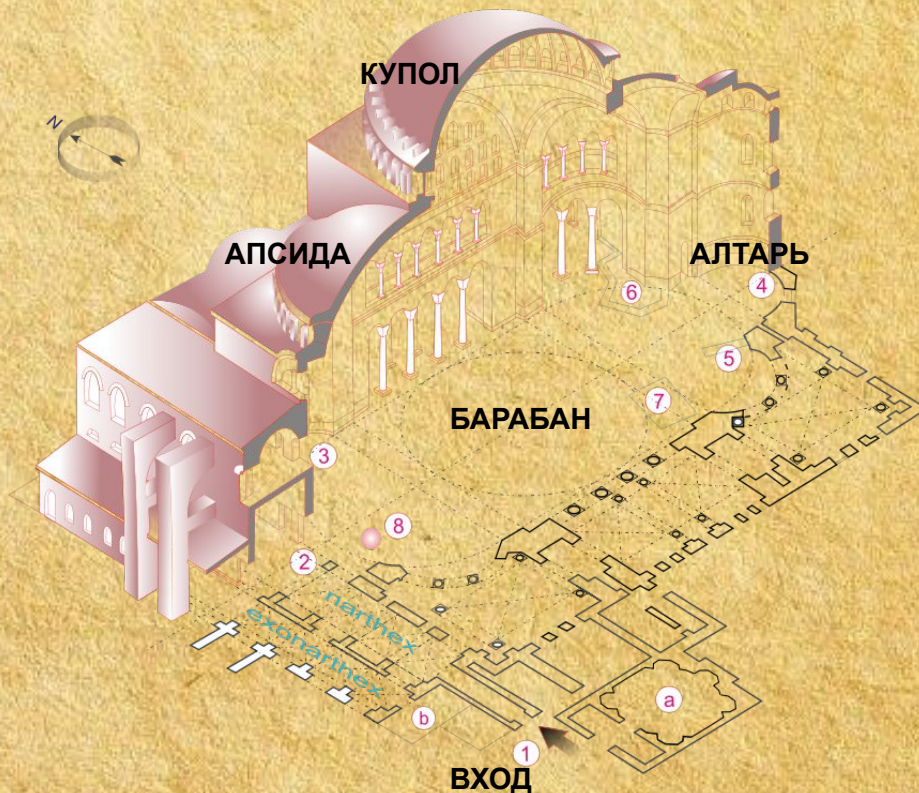
ПЛАН - ХРАМ СВЯТОЙ СОФИИ В КОНСТАНТИНОПОЛЕ ПРИ ЮСТИНИАНЕ
