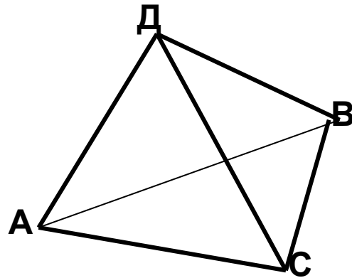
тетраэдр
