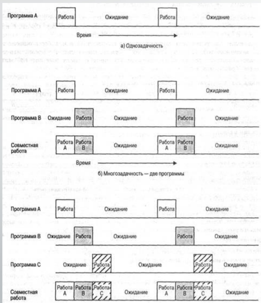
Рис. 2.0 Пример однозадачности и многозадачности.
