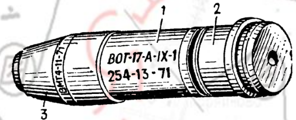
Общий вид выстрела с осколочной гранатой к гранатомету АГС-17 (ВОГ-17): 1 - осколочная граната; 2 - пороховой заряд; 3 - взрыватель
