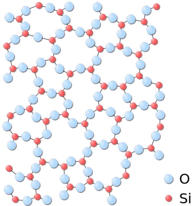
Аморфная структура гладкого кварца ( \text{SiO}_2 )
