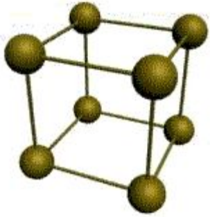
кубическая
