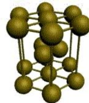
гексагональная плотноупакованная
