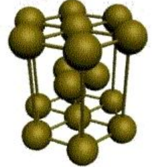
гексагональная плотноупакованная
