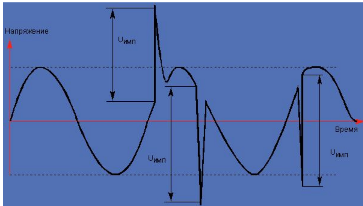
Рисунок 3. Импульсы напряжения.
