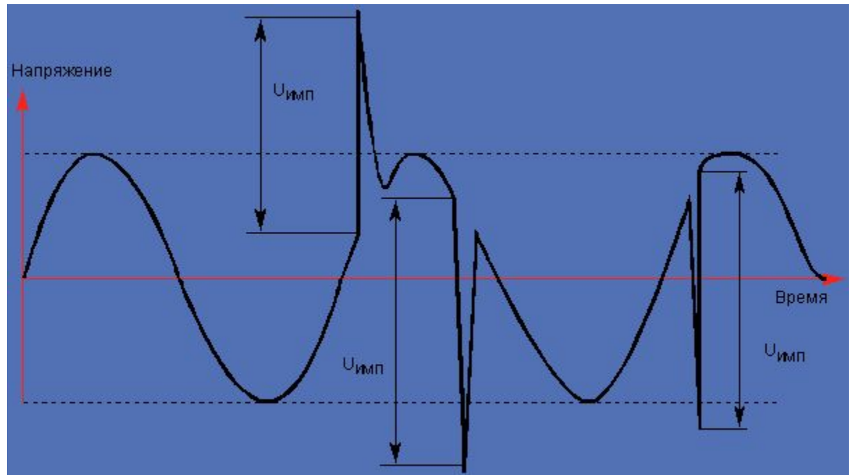
Рисунок 3. Импульсы напряжения.
