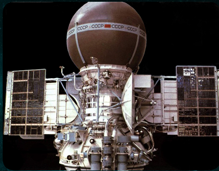
Станция Венера-9
