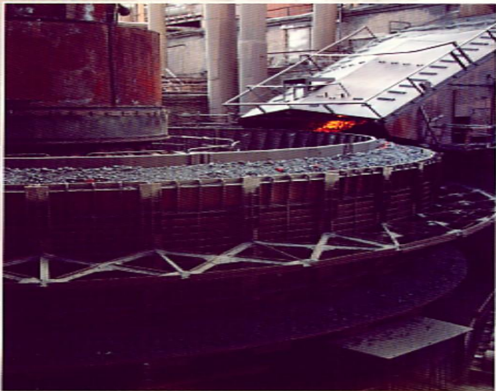
Чашевый охладитель агломерата
