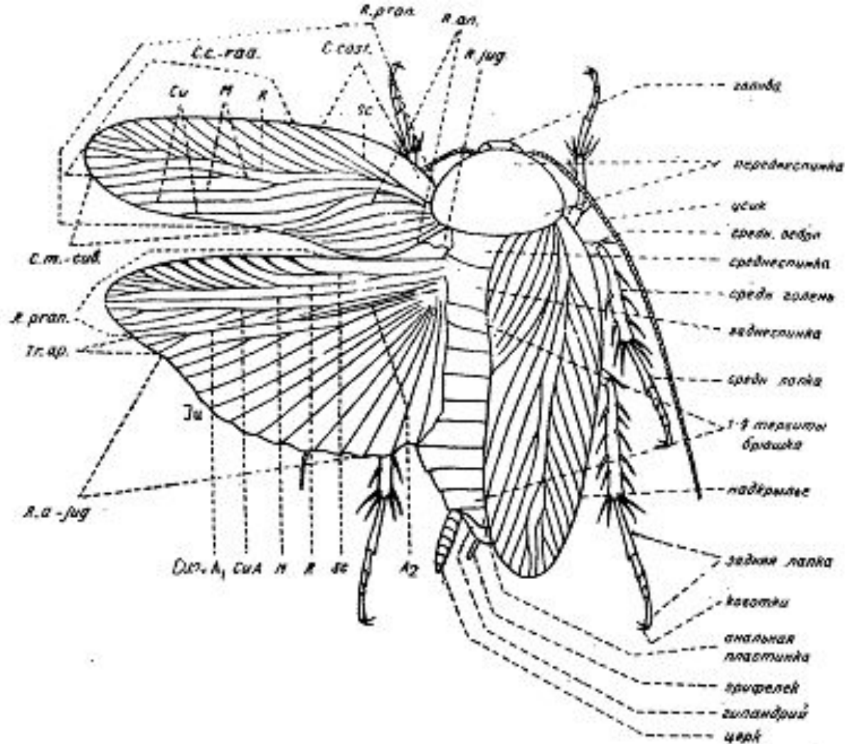
Фиг. 1. Тело таракана сверху. Области крыльев: R. gran. — преданальная область ( regio praeanalis ); R. anal. — анальная область ( r. analis ); R. jug. — югальная область ( r. jugalis ); R. a.-jug. — ано-югальная область ( r. ano-jugalis ). Поля: C. cost. — краевое, или костаальное, поле ( campo costalis ); C. s.-rad. — косто-радиальное поле ( c. costo-radialis ); C. t.-sub. — медио-кубитальное поле ( c. medio-cubitalis ); Tr. ap. — верхний треугольник ( triangulus apicalis ). Жилки: Sc — субкоста; R — радиус; M — медиана; Cu — кубитус; CuA — кубитус передний; CuP — кубитус задний; A 1 — анальная первая; A 2 — анальная вторая; Ju — югальные. Ориг.
