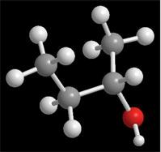
Бутанол -2
