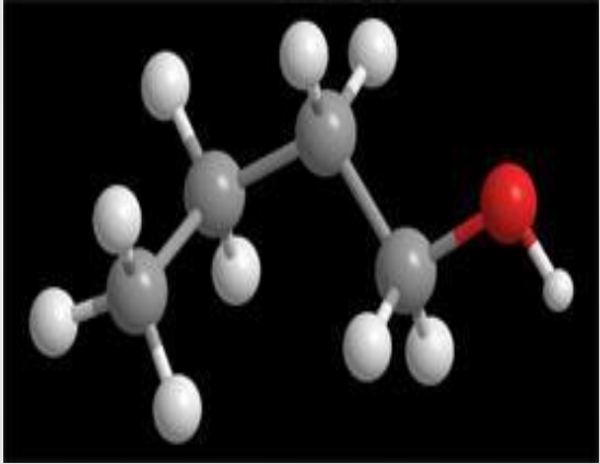
Бутанол -1
