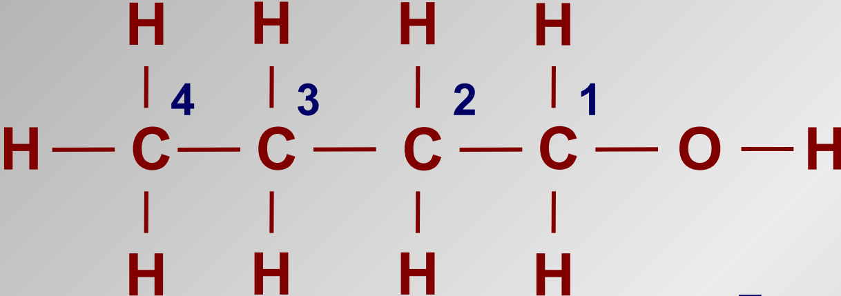
Бутанол -1
