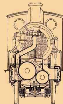
Черт. 6. Компаунд-паровоз Воределя (Worsdell).
