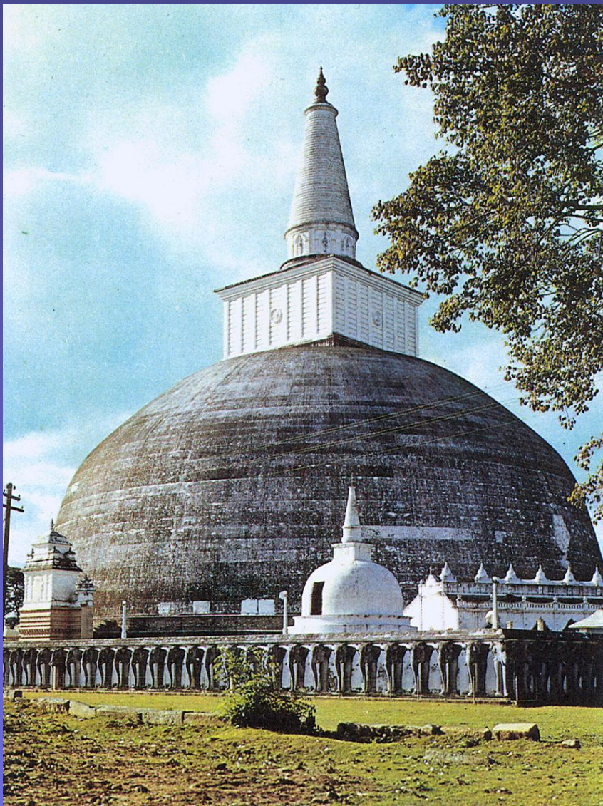
Ступа Шри-Ланки
