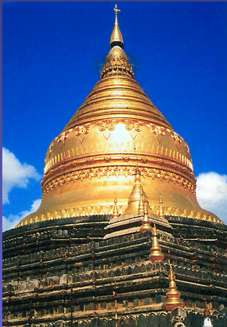
Ступы Бирмы
