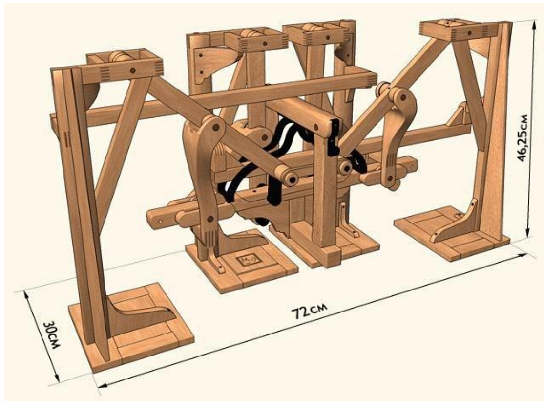
Стопоходящая машина (1878)
