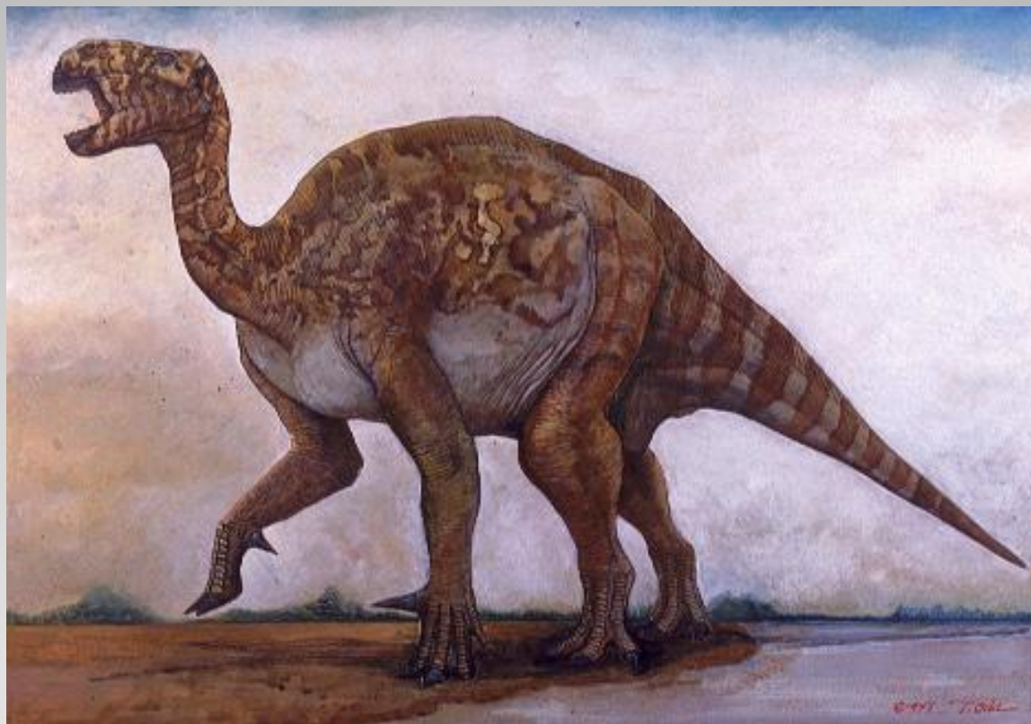
Игуанодон.
