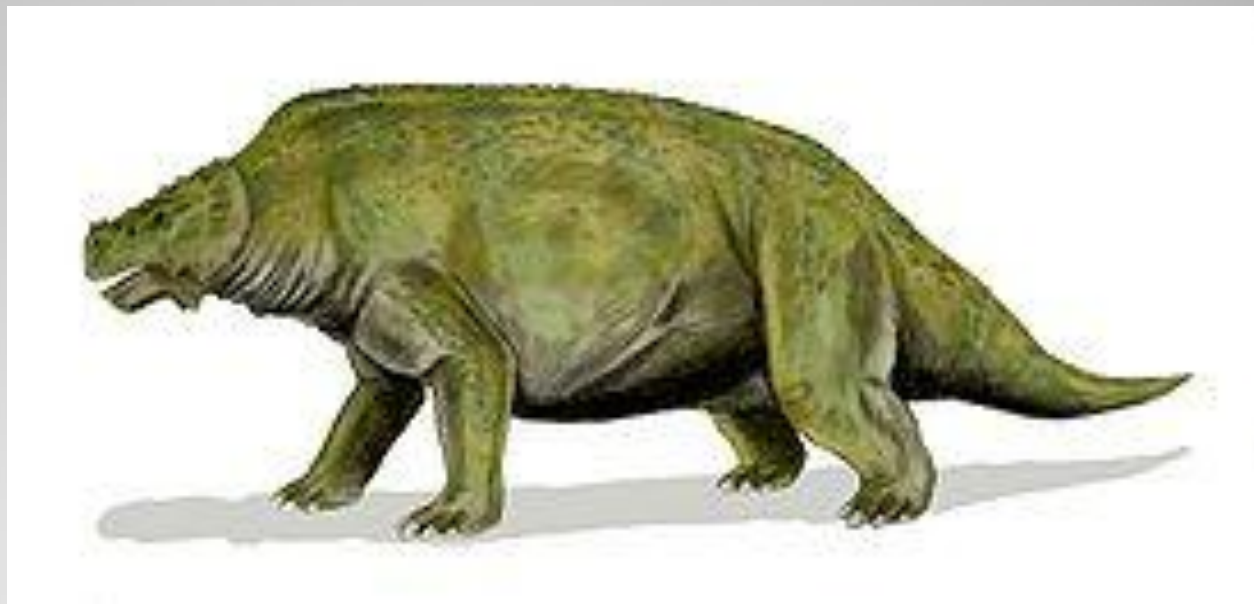
Парейазавр.
