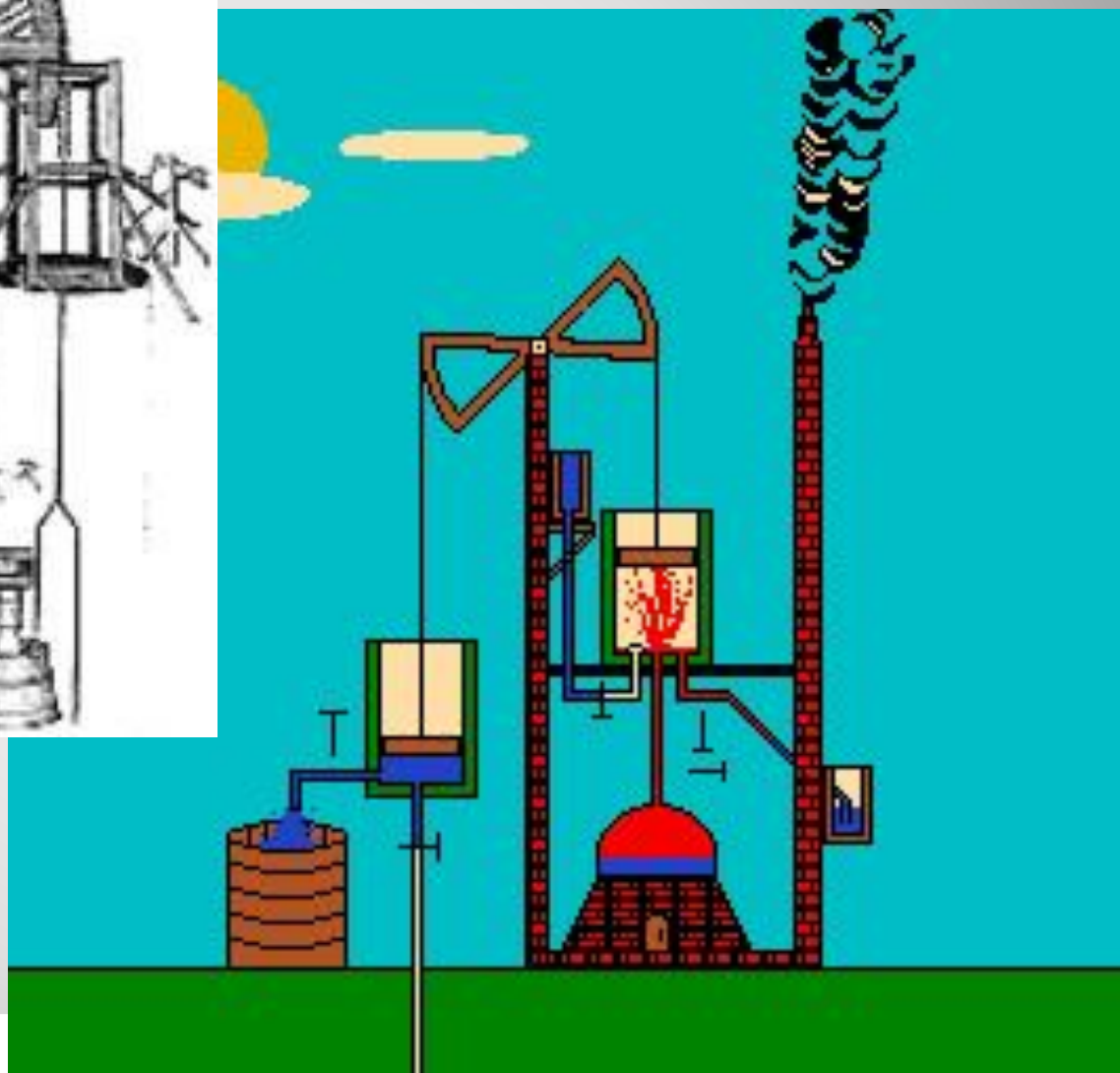
Принцип работы машины Ньюкомена
