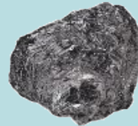
Галенит
