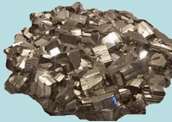
Пирит
