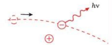
Механизм возникновения тормозного рентгеновского излучения
