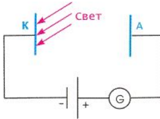
Схема экспериментальной установки для изучения фотоэффекта
