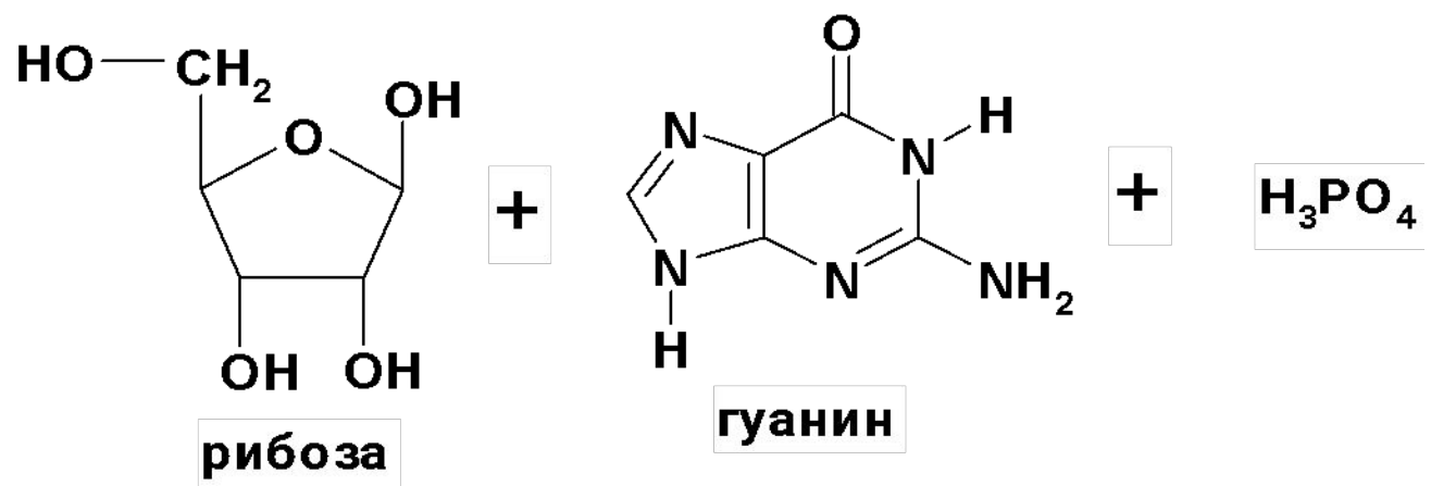
гуанозин-5'-фосфат
