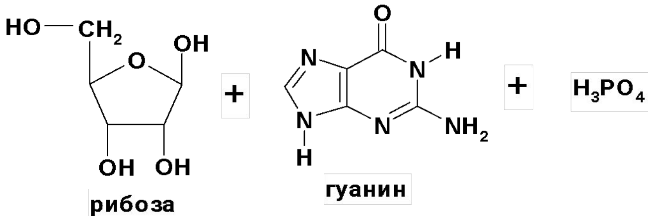
гуанозин-5'-фосфат
