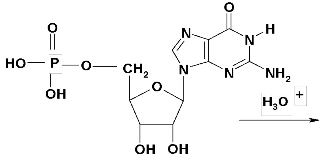
гуанозин-5'-фосфат
