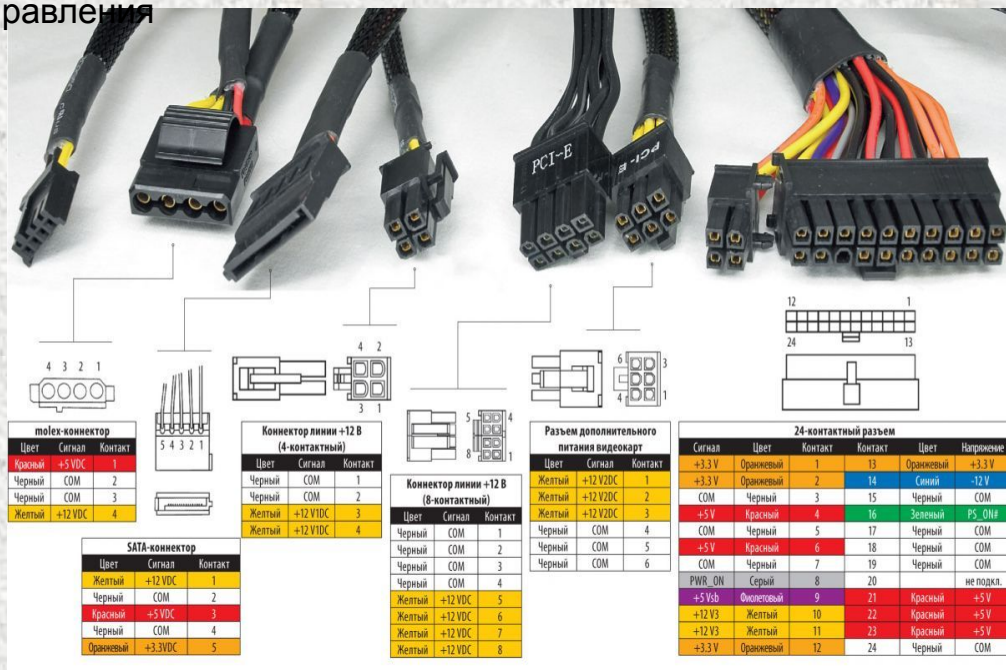
На данном рисунке показана распиновка контактов блоков питания, традиционно используемых в современных ПК
