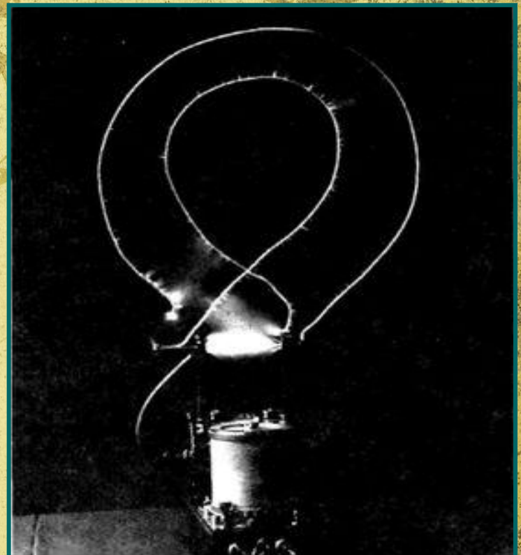
Колебательный контур
