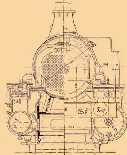
Черт. 6. Компаунд-паровоз Воределя (Worsdell).
