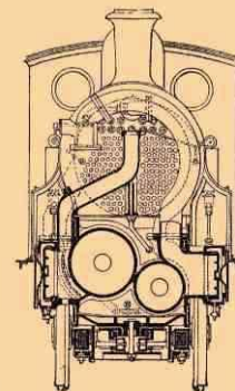
Черт. 6. Компаунд-паровоз Воределя (Worsdell).
