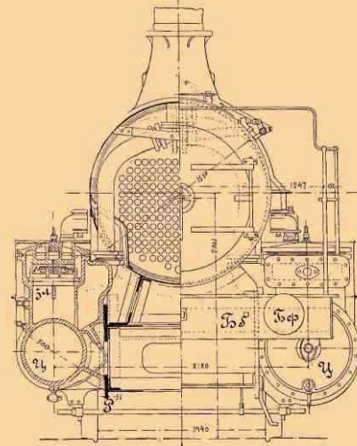
Черт. 6. Компаунд-паровоз Воределя (Worsdell).
