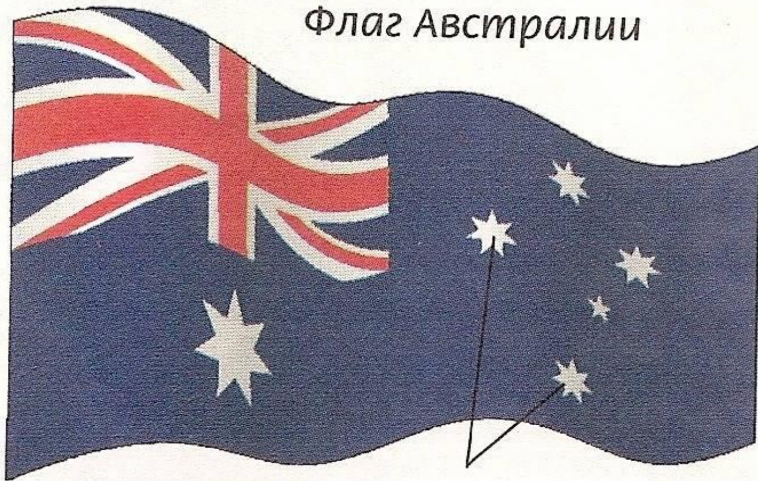
Созвездие Южного Креста
