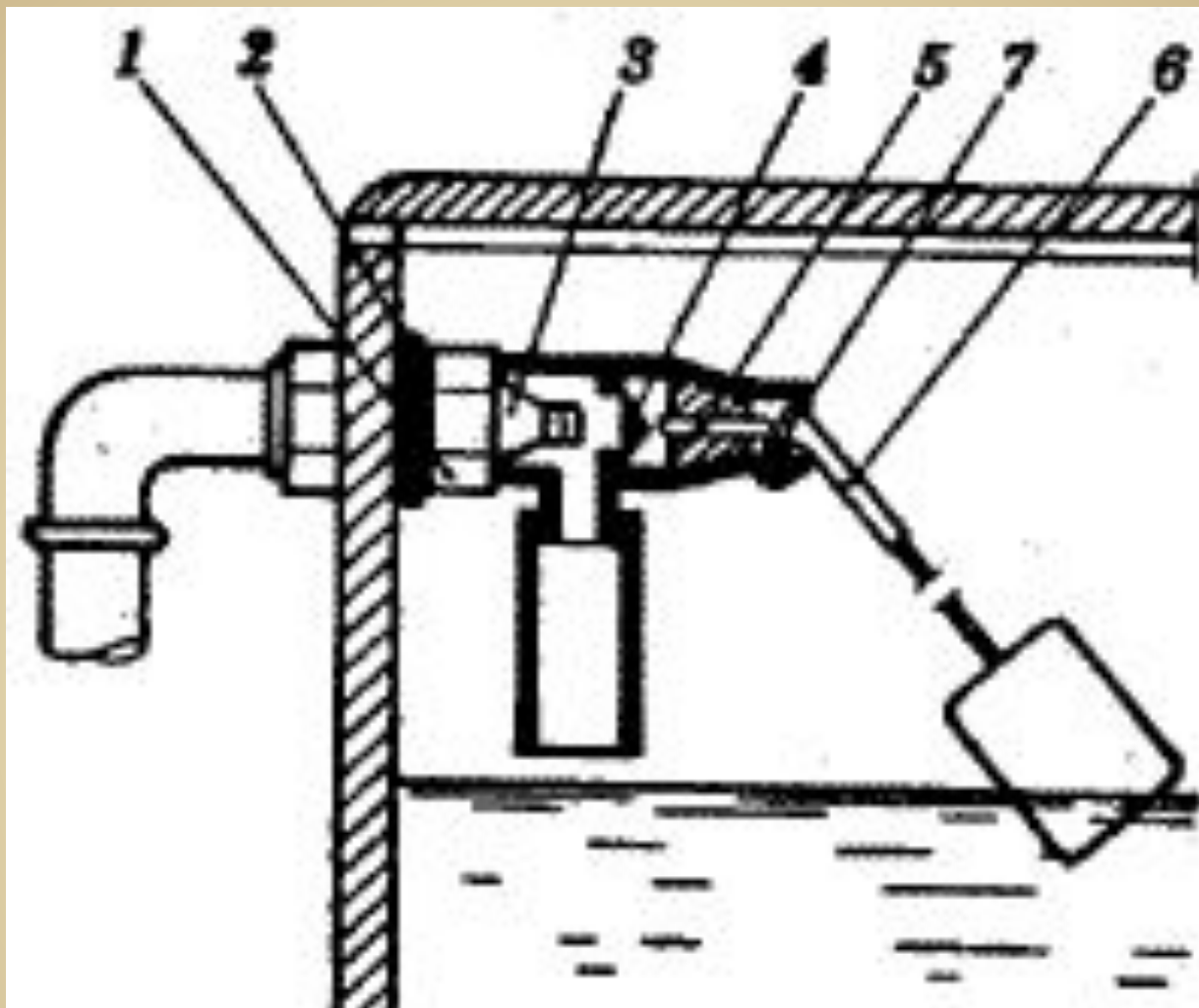
Поплавковый клапан - конструкция: 1 - прижимная шайба; 2 - прокладка; 3 - седло; 4 - мембрана; 5 - стержень; 6 - рычаг поплавка; 7 - ось рычага.
