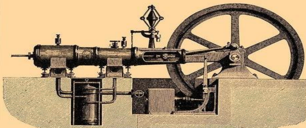
2. Горизонтальная паровая машина Вулфа.
