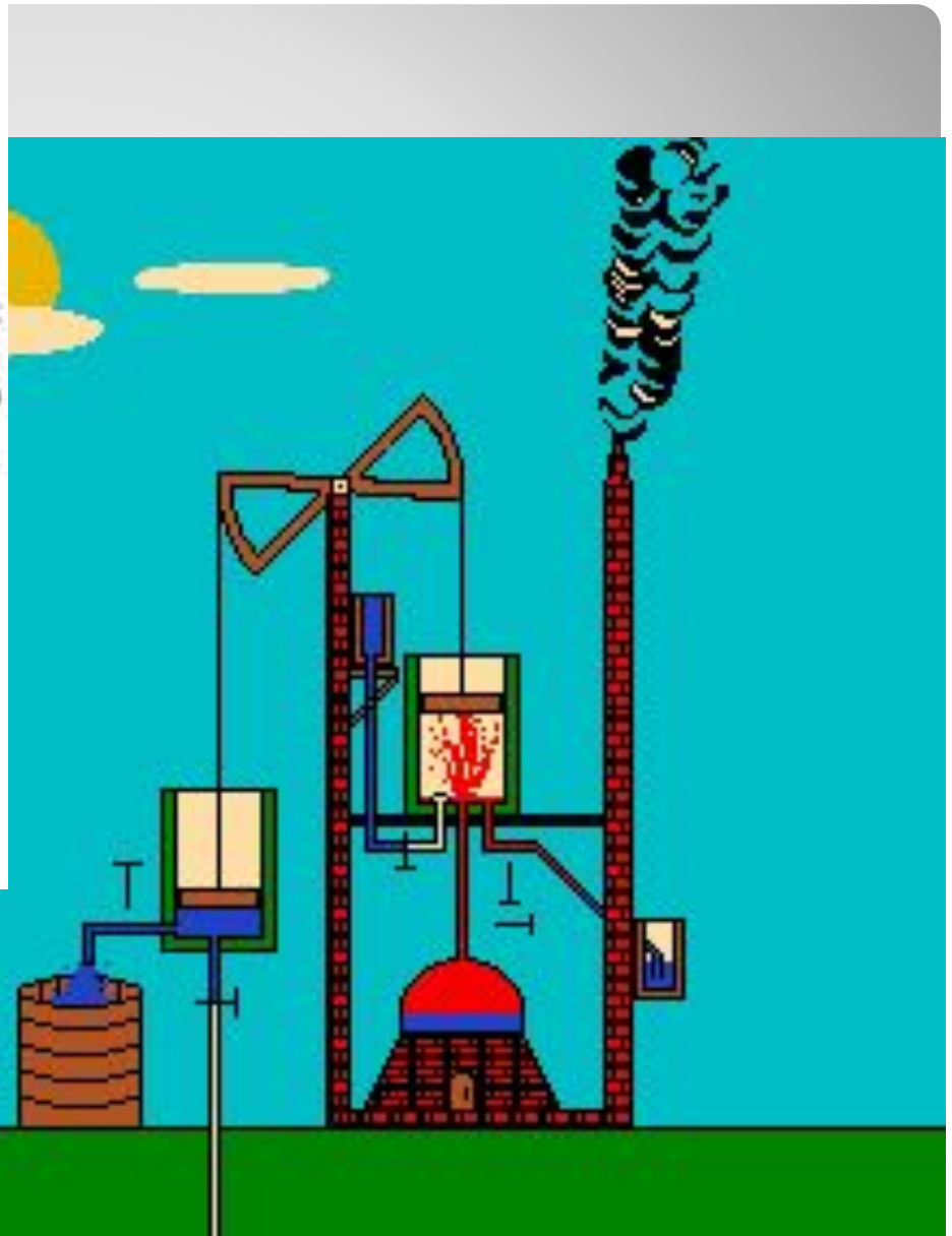
Принцип работы машины Ньюкомена
