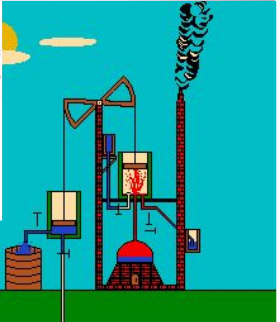
Принцип работы машины Ньюкомена
