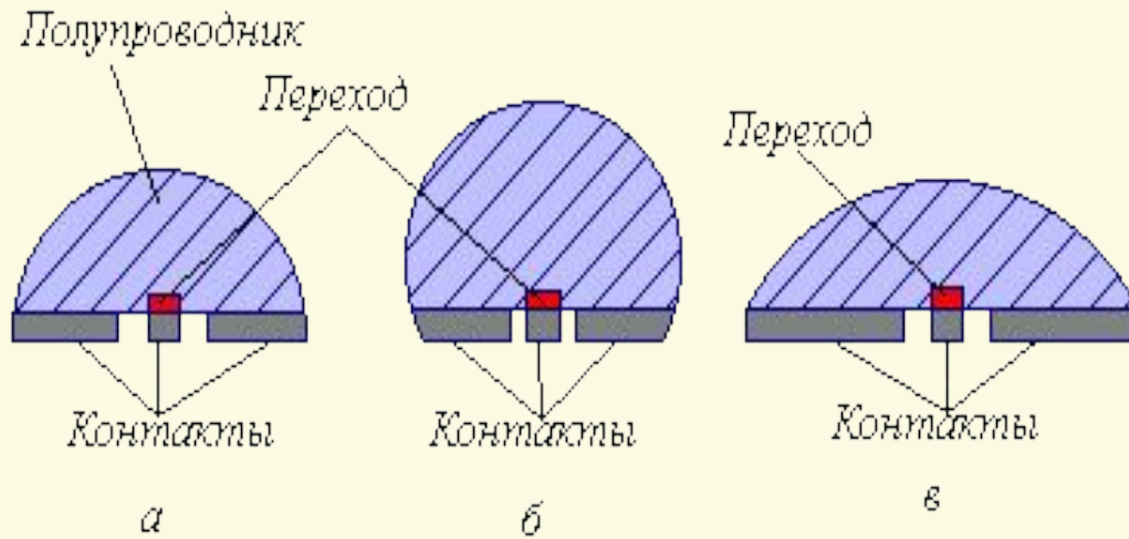
а-полусфера; б-усечённая сфера; в-параболоид
