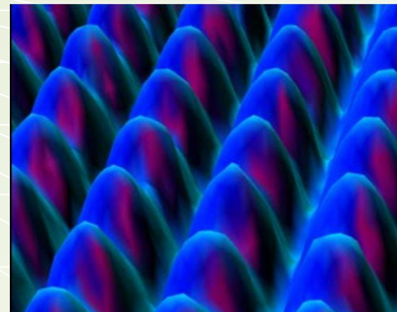
Атомы никеля
