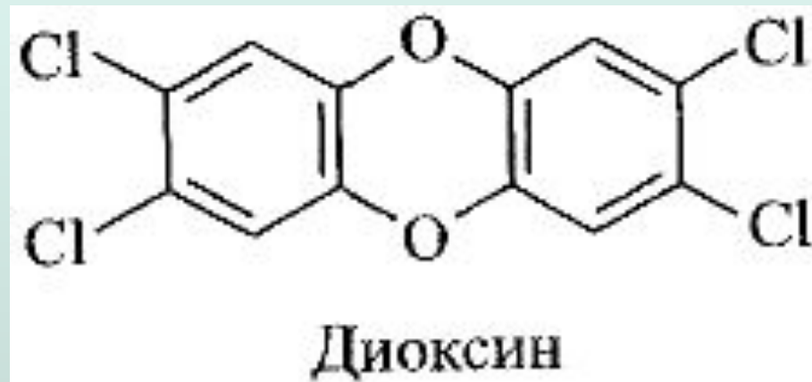
Диоксин 2,3,7,8-тетрахлордibenзо-p-диоксин
