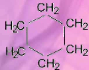
Циклогексан
