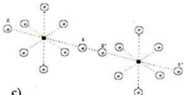
Молекула кислорода
