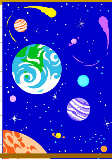
Гелиоцентрическая система
