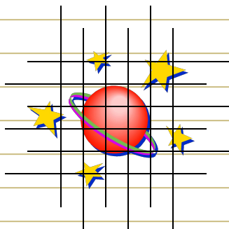
Геоцентрическая система
