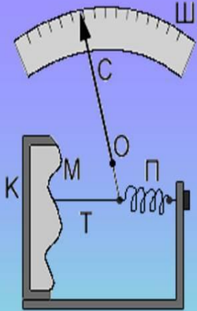
Схема барометра - анероида
