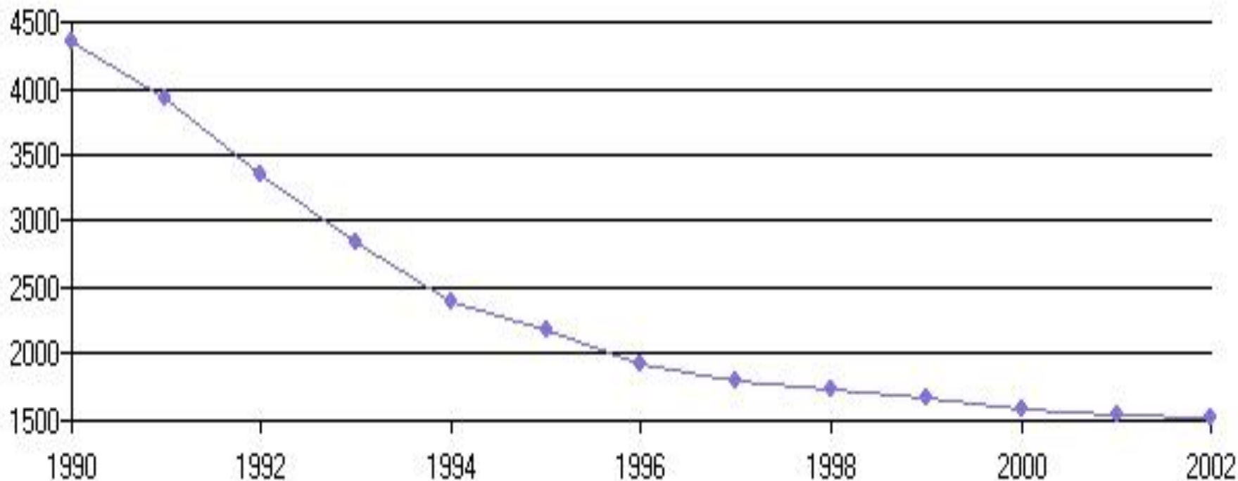
Выбросы загрязняющих веществ в атмосферу (тыс. т)
