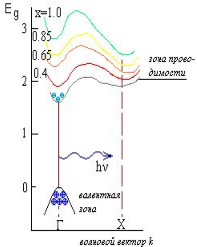
Энергетическая зонная структура \text{GaAs}(1-x)\text{P}(x) Значения состава соответствуют красному ( x=0,4 ), оранжевому ( 0,65 ), жёлтому ( 0,85 ) и зелёному свету ( 1,0 )
