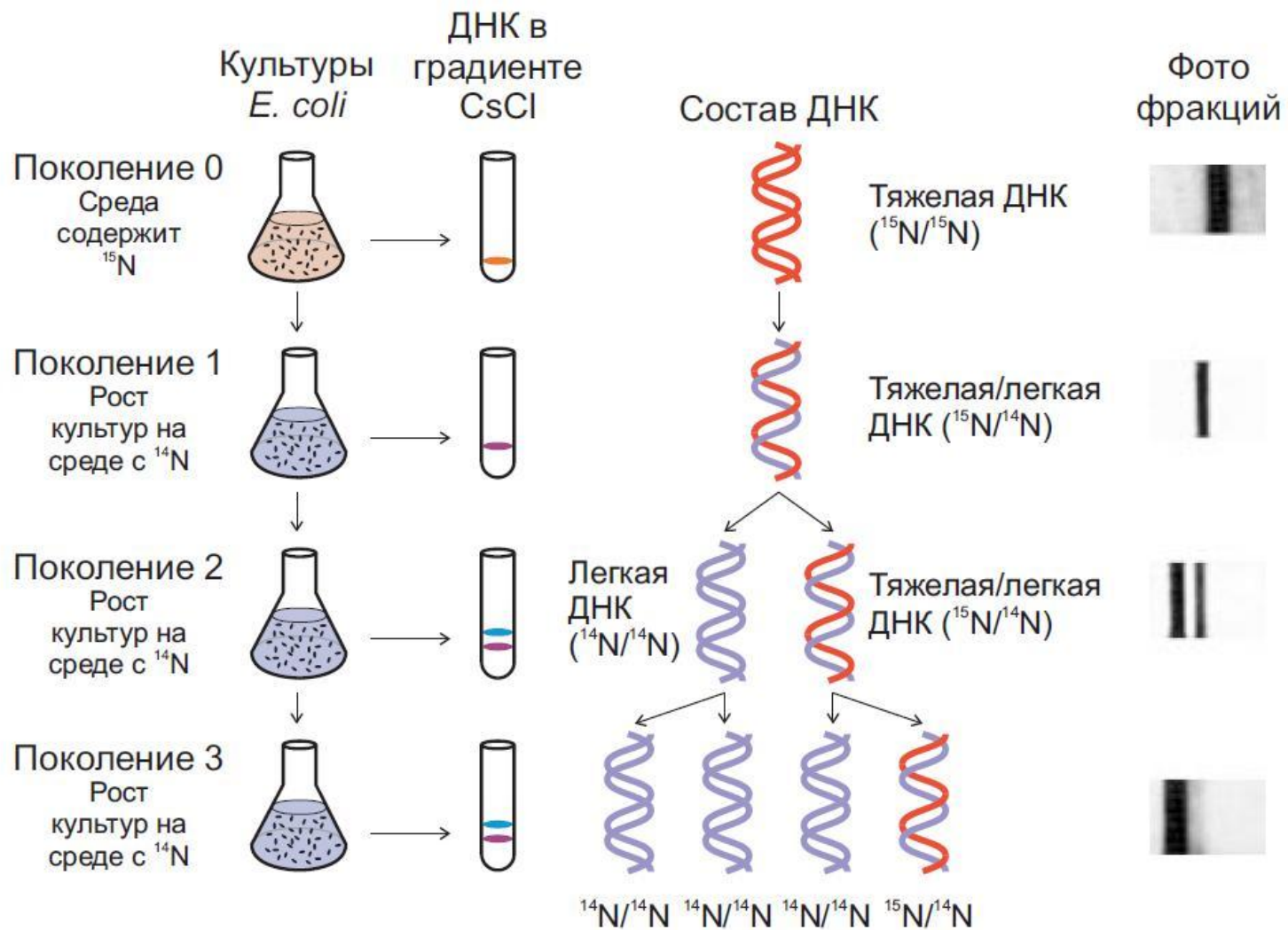
Схема опытов Мезелсона и Сталя, доказывающих полуконсервативную модель репликации ДНК (Из: Russell, 1998, p. 346).
