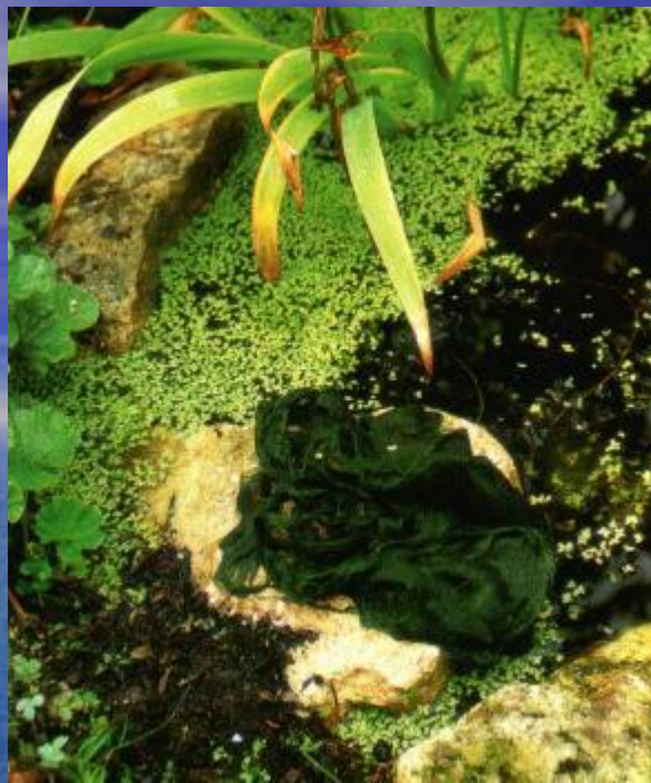
Водоросли спиругира
