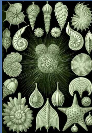
раковины фораминифера
